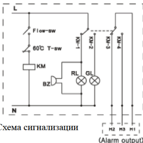
Выходы сигнализации
